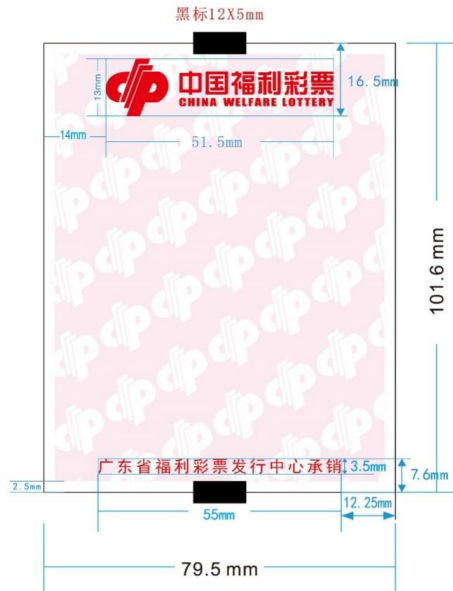
图1 固定长度票面版式要求示意图
